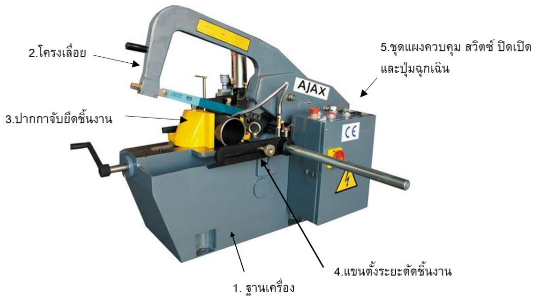
รูปที่ 1-2 ส่วนประกอบของเครื่องเลื่อยกลแบบชัก
