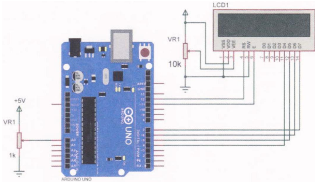
รูปที่ 8.8 วงจรการทดลองโปรแกรมแปลงอนาล็อกเป็นดิจิทัลแสดงผลจอ LCD
