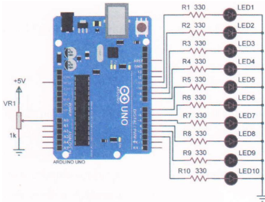
รูปที่ 5.7 วงจรการทดลองโปรแกรมการอ่านค่าอนาล็อกแสดงผลที่หลอดแอลอีดี
