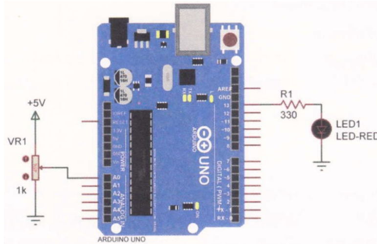
รูปที่ 8.6 วงจรโปรแกรมไฟกะพริบตามคววนาล็อกอินพุต
