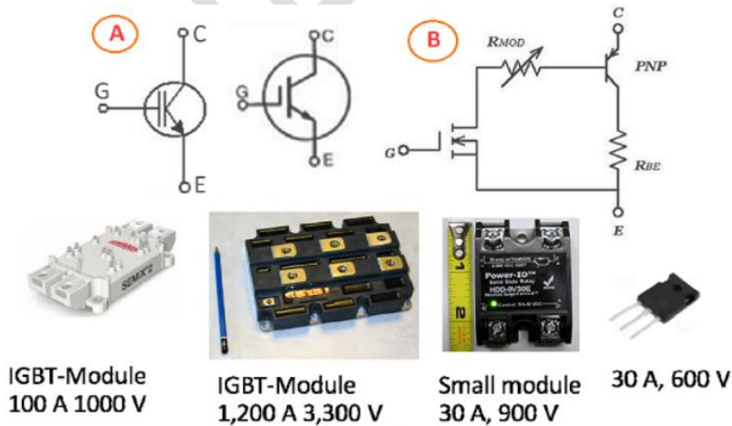
รูปที่ 1 สัญลักษณ์ไอบีจีที(IGBT)
