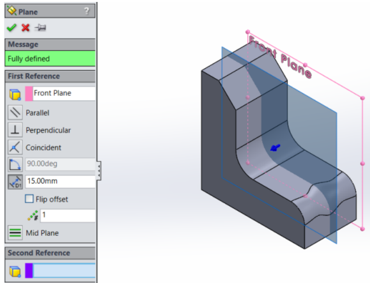
รูปที่ 16 : การสร้างระนาบ Plane เพื่อกำหนดพื้นที่ของโครงสร้าง
