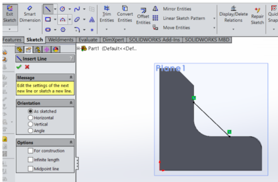
รูปที่ 17 : การสร้างเส้นเชื่อมระหว่างระนาบทั้งสองที่ตั้งฉากกัน
