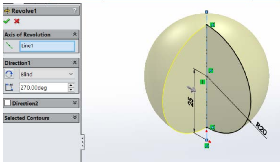
รูปที่ 3 : กำหนดองศาการหมุนในคำสั่ง Revolved Boss/Base
